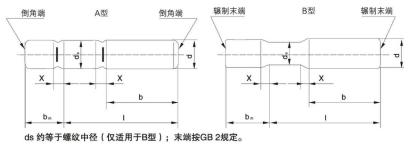
ds 约等于螺紋中径 (仅适用于B型); 束端按GB 2规定。
